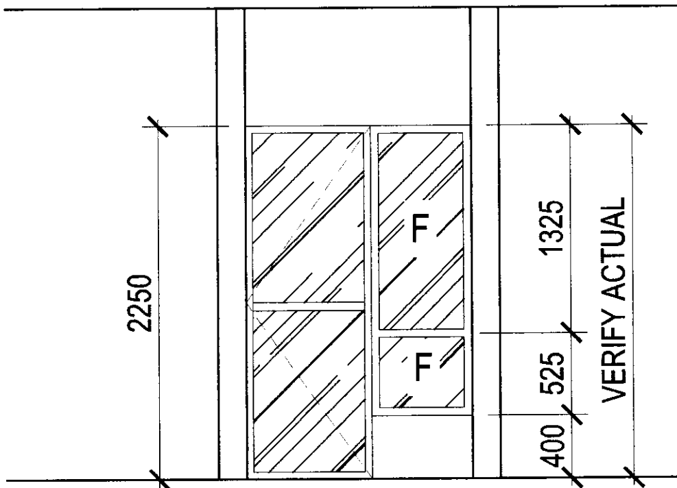
ELEVATION
